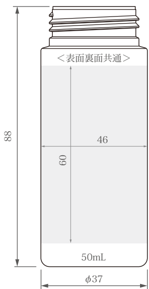
PF-50 材質：HDPE+バイオマスPE ※ 成形方法：ダイレクトブロー
