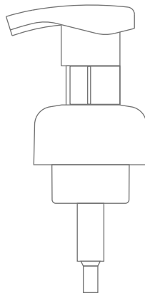
F6 ポンプフォーマー 吐出量：0.75cc (受注対応品)
